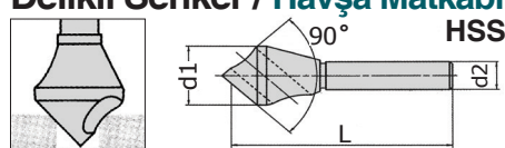
90° HSS Delikli Senker / Havşa Matkabı
