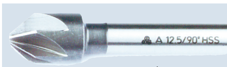
90° HSS Çok Ağızlı Havşa Matkabı
