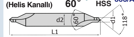
60° HSS 333/A Uzun Punta Matkap Ucu (Helis Kanallı)
